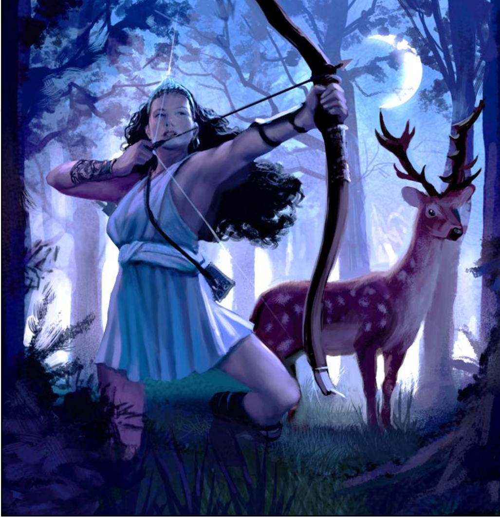
Şekil 43: Artemis illüstrasyonu 104
