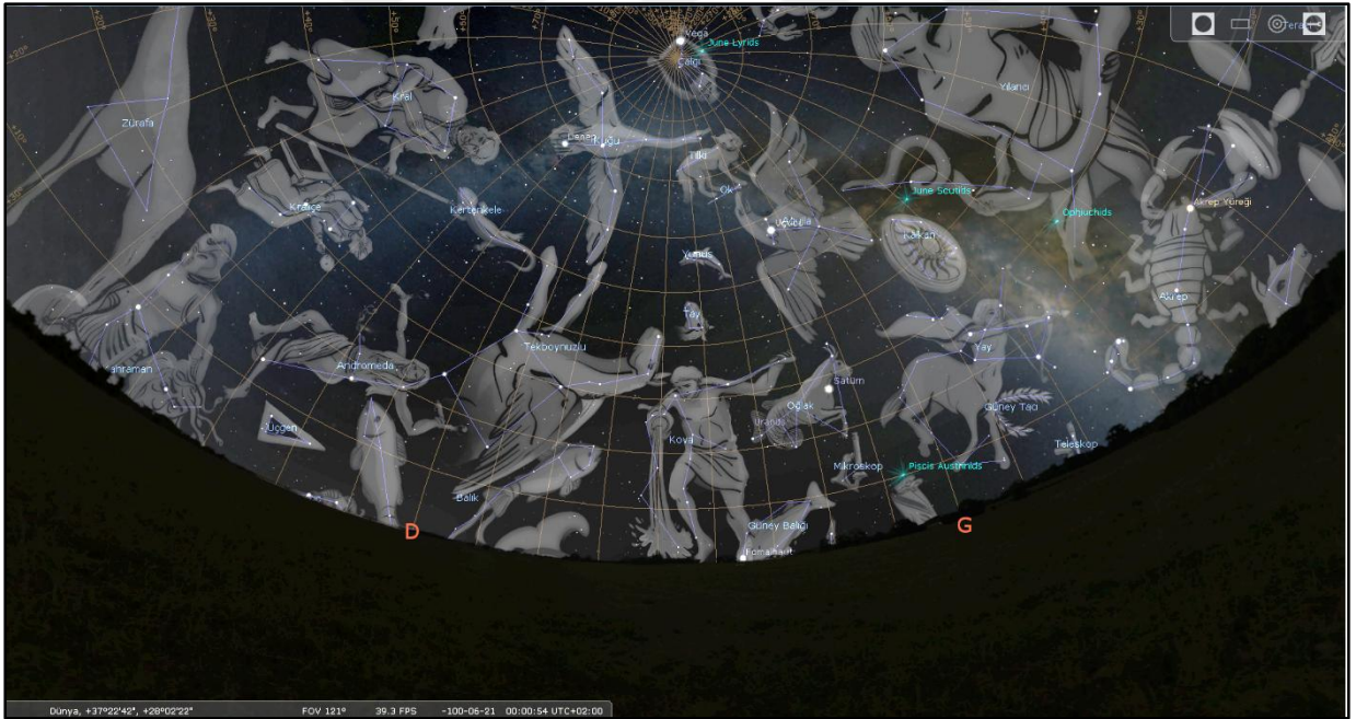
Şekil 107: Hekate Tapınağı (Tarih: 21 Haziran, MÖ 100) (Yön: Güneydoğu) (Program: Stellarium)
